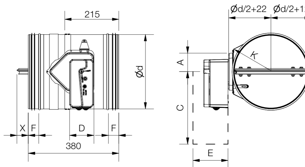
FDC40-R40 (d355 do d800)
